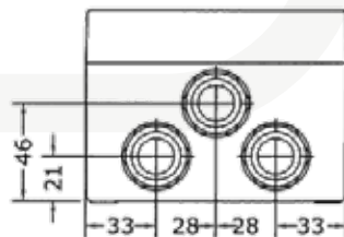
Side B: 3 cable glands M25x1,5 blue
